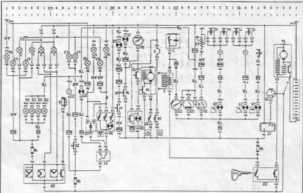
SCHEMA DE PRINCIPE DES CITROEN Méhari
