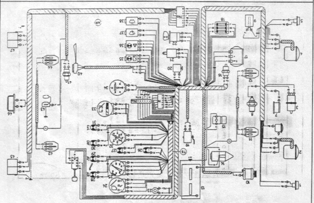
SCHEMA ELECTRIQUE DES CITROEN Méhari
