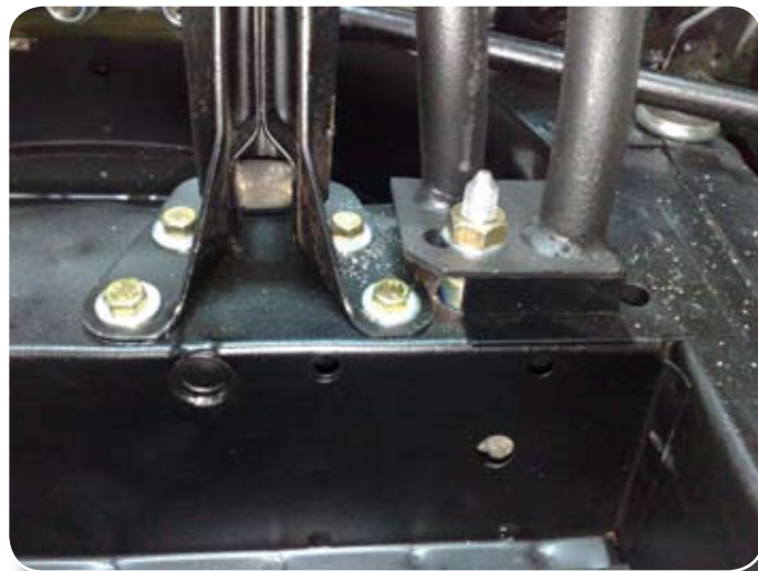
Vue fixation gauche
